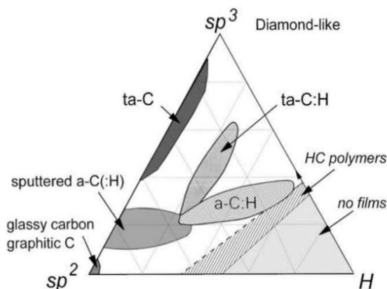
FIGURA 2: Diagrama de fase ternária das ligações em ligas de carbono amorfo hidrogenado.
