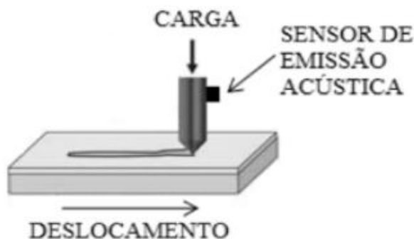
FIGURA 3: Representação do Ensaio de Riscamento. Fonte: Costa, 2010
